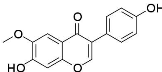
(d) Glycitein
